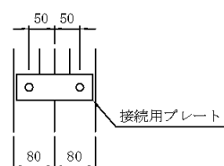
ジョイント部詳細図
