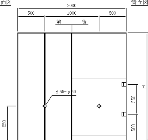
正面図
