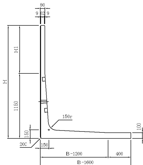
側面図
