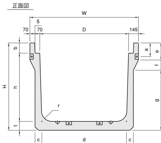
W X 側溝寸法重量表 内空高さ h=700
