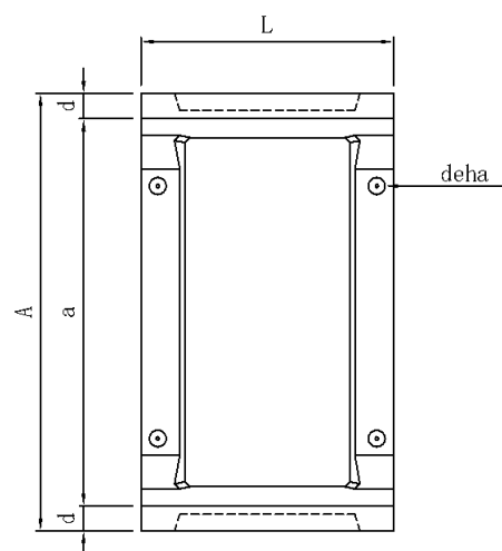
h=2100用 寸法・重量表
