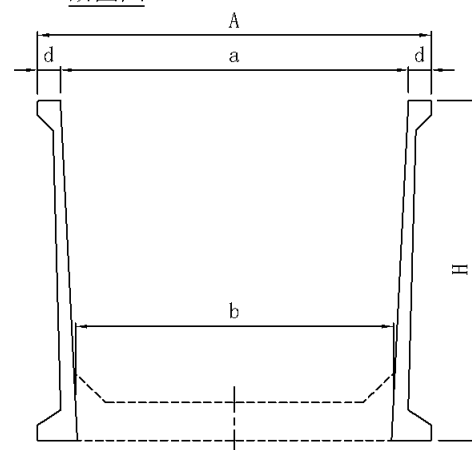
断面図
