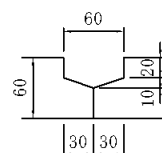
ジョイント部詳細
