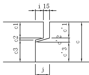
ジョイント部詳細図
