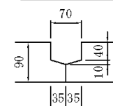
ジョイント部詳細
