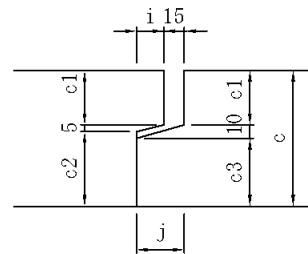
ジョイント部詳細図
