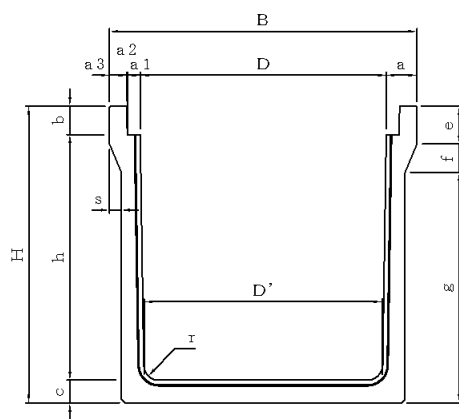
寸法表 (h-1300型)
