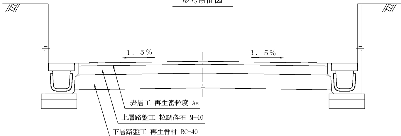
参考断面図
