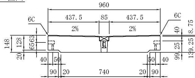
正面図
