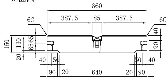
正面図
