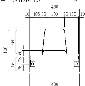
出入り口（端末型、反射鏡付き） W=513kg
