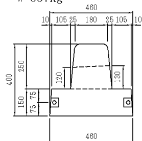
出入り口（平型） W=343kg
