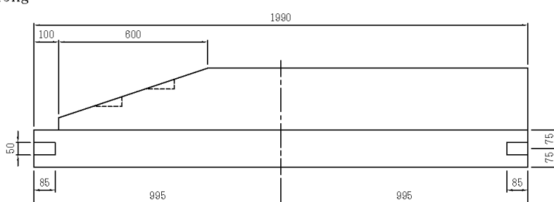
ジョイント部詳細
