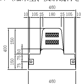
出入り口（端末型、反射鏡付き） W=513kg
