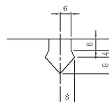
目地部詳細図
