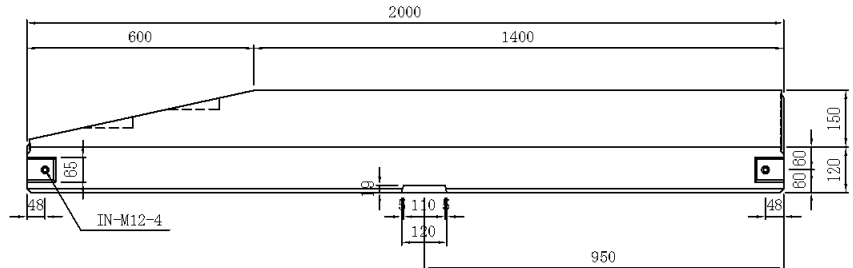
目地部詳細図
