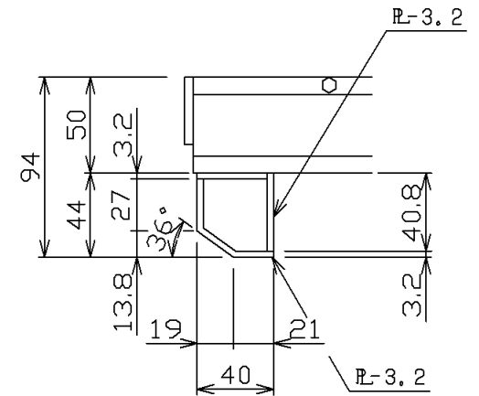
詳細 "A"
