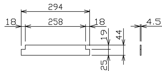
FB4.5X44 (止メ) 詳細
