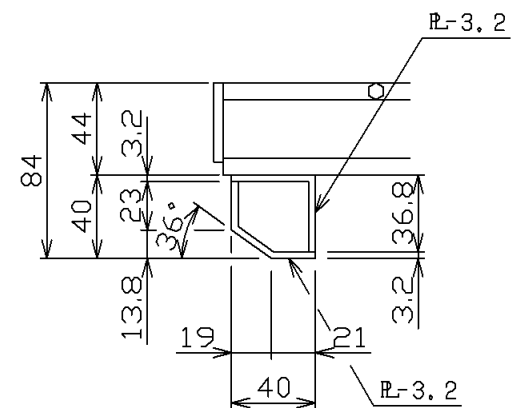
詳細“A”
