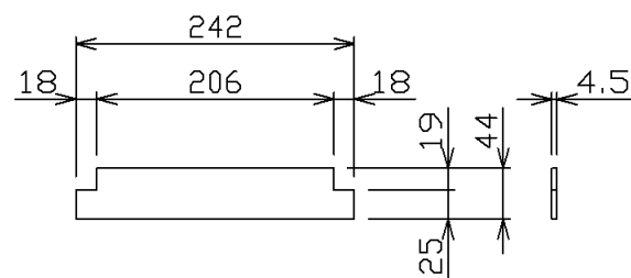
FB4, 5X44 (スレ止め) 詳細
