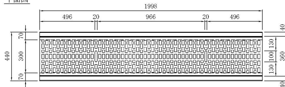
平面図
