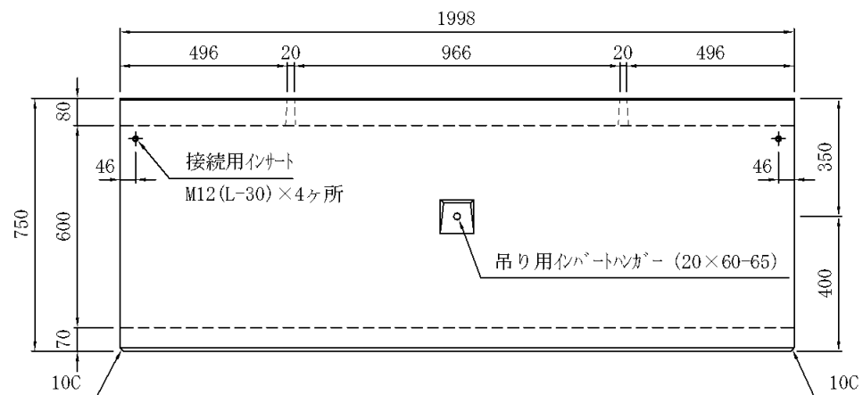
側面図
