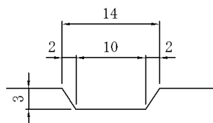
シーリング目地詳細図
