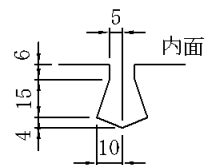
目地部詳細図
