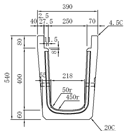
構造図
