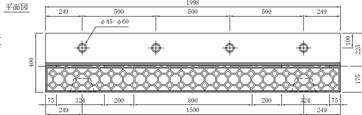
スリット部詳細図
