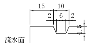
本体目地詳細図
