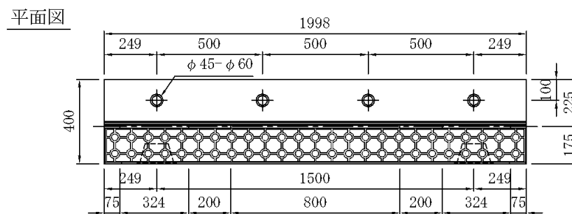
スリット部詳細図
