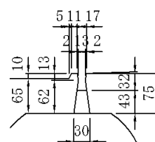
スリット部詳細図
