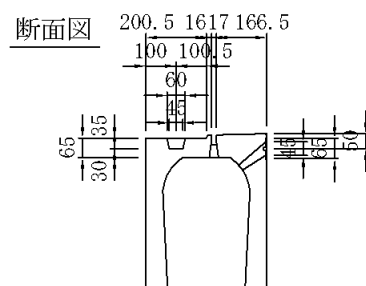
フランジ詳細図
