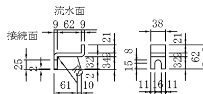
フランジ詳細図
