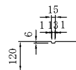
スリット部詳細図
