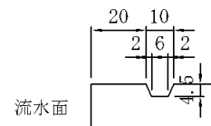
本体目地詳細図
