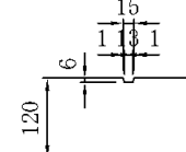
スリット部詳細図
