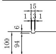
スリット部詳細図
