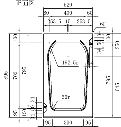
正面図
