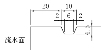
本体目地詳細図
