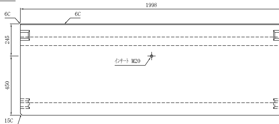
側面図
