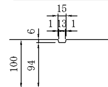
スリット部詳細図
